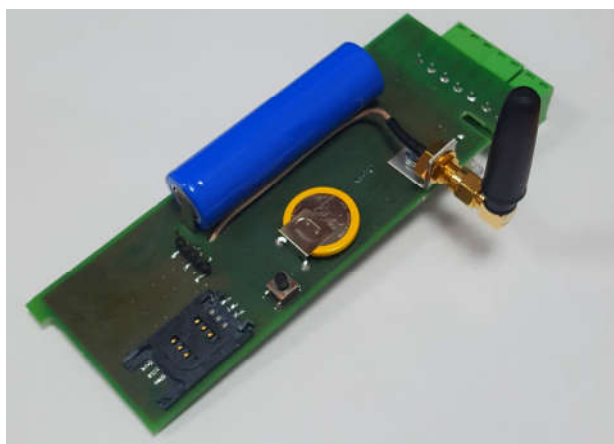
Плата извещателя вынута из корпуса: синего цвета – буферный аккумулятор, желтого цвета – батарейка часов, крепление SIM-карты – в углу платы
